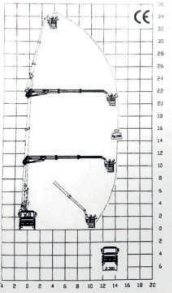
Diagramma di lavoro in sagoma : piazamento 2300 mm
